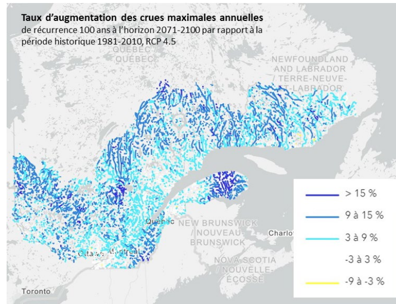
Source graphique : Atlas hydroclimatique du Québec méridional
